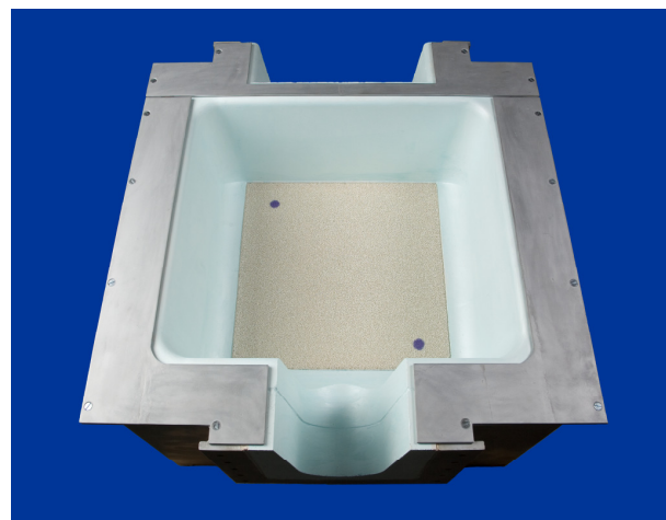
Двухступенчатая чаша SELEE® с двумя фильтрами
