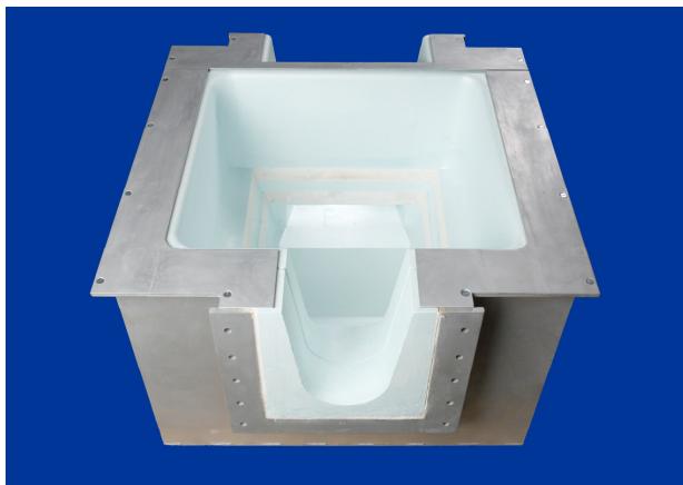
Двухступенчатая чаша SELEE® перед установкой фильтров
